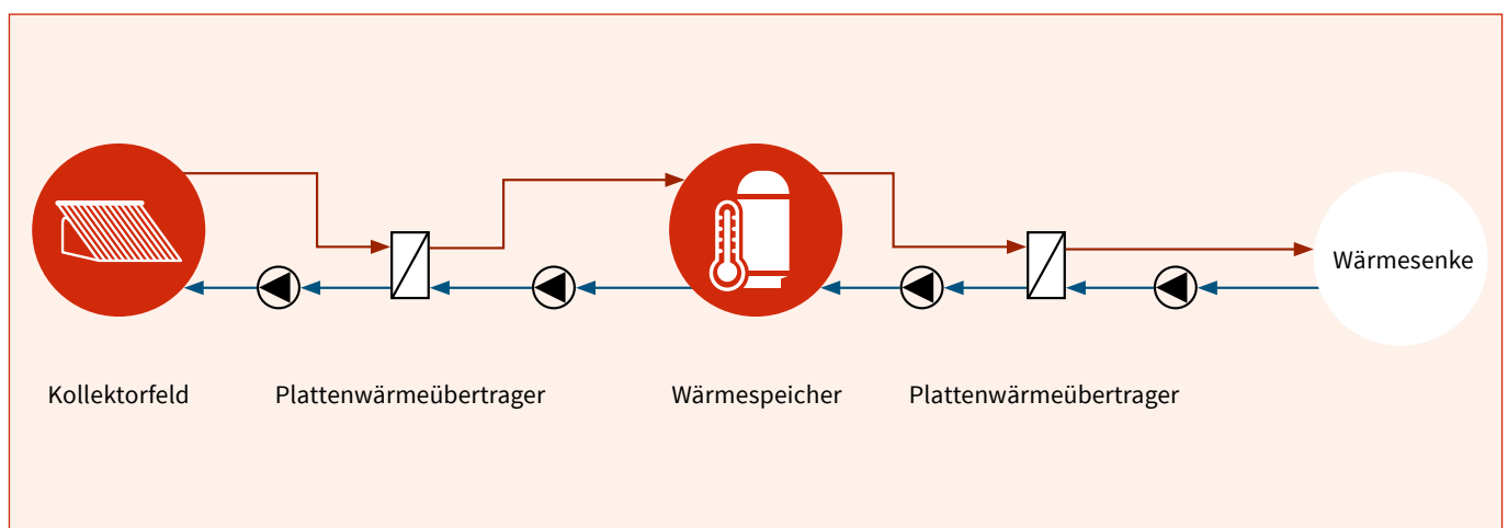
Abbildung 2: Vereinfachtes Hydraulikkonzept einer solaren Prozesswärmeanlage mit deren Hauptkomponenten.
