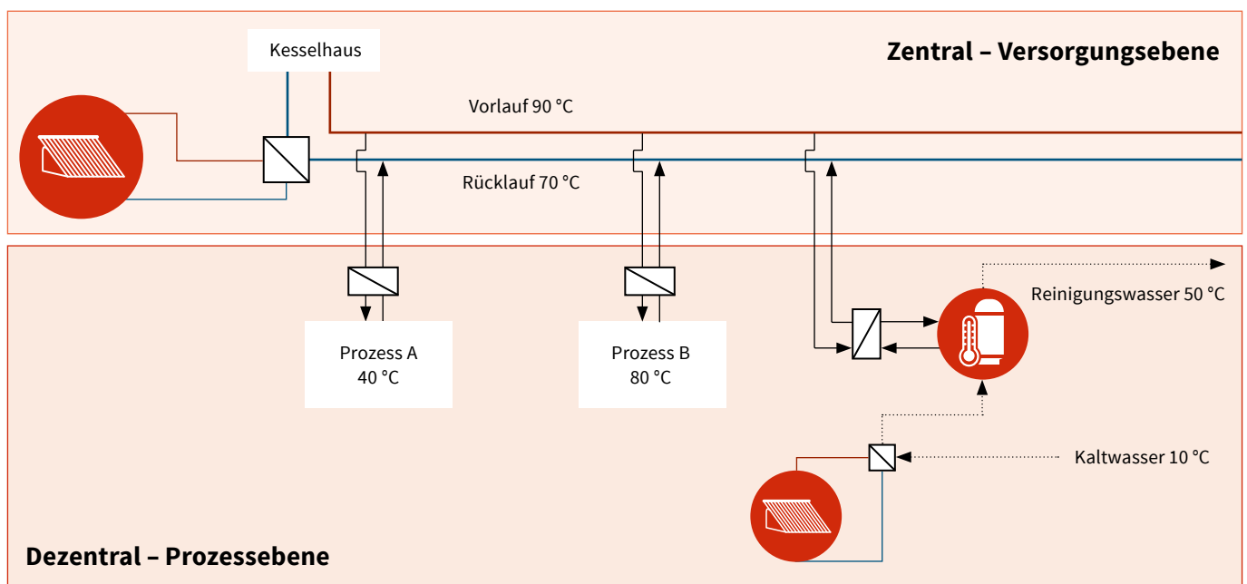
Abbildung 3: Einbindungsmöglichkeiten solarer Prozesswärmeanlagen in die Prozesse.
